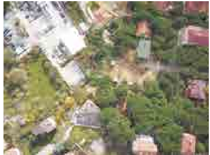
Şekil 7: Pervaneli İnsansız Hava Aracı ile çekilen bir ortofoto örneği
