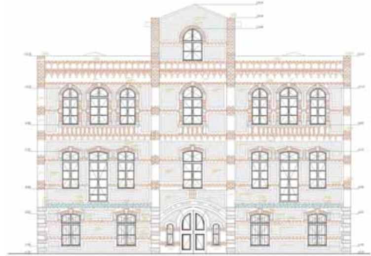
ÖN CEPHE ÖLÇEK: 1/ 50
