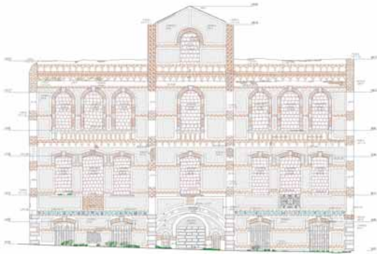
ÖN CEPHE ÖLÇEK: 1/ 50
