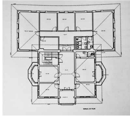
Zemin kat planı (sol), 1. kat planı (sağ)
