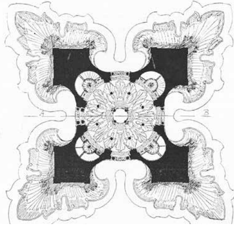
Kulenin üçüncü kattan görünüşü (sol), Kulenin zemininden görünüşü (sağ)
